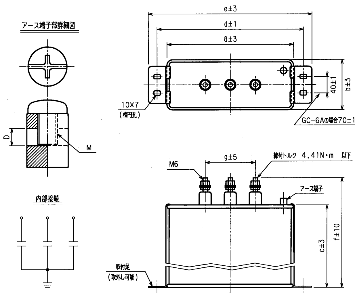
GC-4A, 5A, 6A 外形図・寸法表
