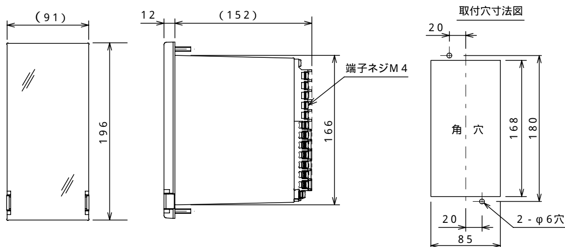
角胴ケース 外形図、取付穴寸法図 (樹脂ケース)
