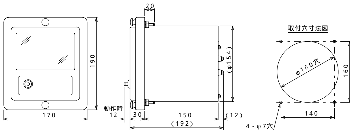
丸胴ケース 外形図、取付穴寸法図
