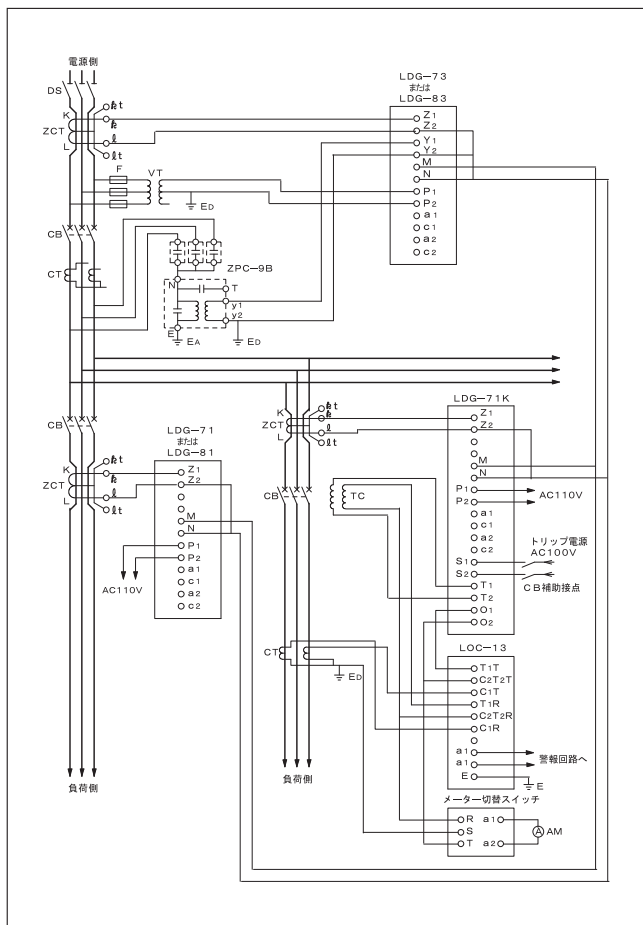
多分岐回路
